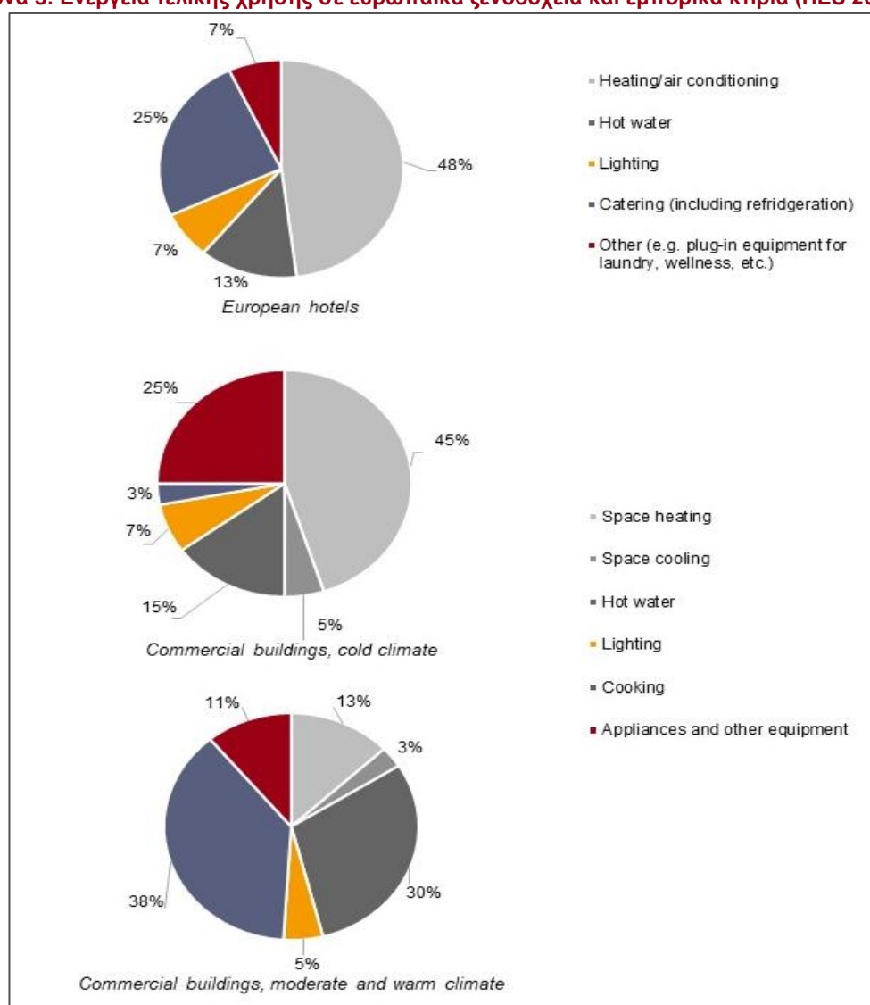
Εικόνα 3: Ενέργεια τελικής χρήσης σε ευρωπαϊκά ξενοδοχεία και εμπορικά κτίρια (HES 2011 and World
