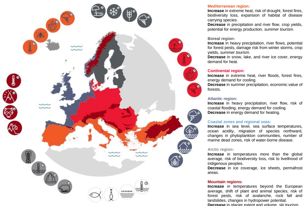
Εικόνα 2: Επιπτώσεις της κλιματικής αλλαγής στις περιφέρειες της Ευρώπης (Ευρωπαϊκός Οργανισμός Περιβάλλοντος [EOX] 2017)
