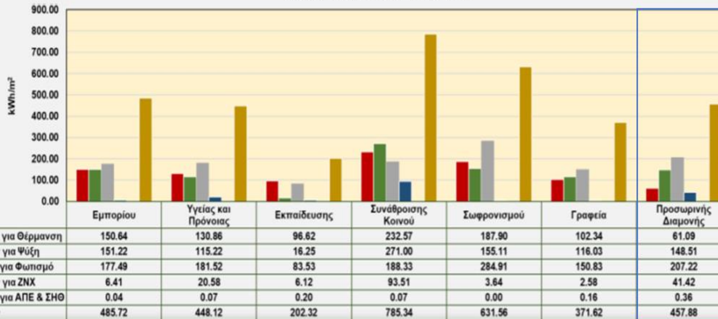
ΜΕΣΗ ΕΤΗΣΙΑ ΚΑΤΑΝΑΛΩΣΗ ΠΡΩΤΟΓΕΝΟΥΣ ΕΝΕΡΓΕΙΑΣ ΚΤΙΡΙΩΝ ΤΡΙΤΟΓΕΝΟΥΣ ΤΟΜΕΑ ΧΡΟΝΙΚΗΣ ΠΕΡΙΟΔΟΥ 2011 -2019
